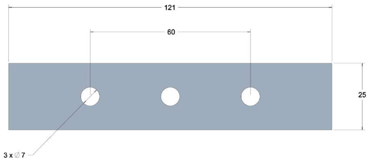
Montážní otvory
