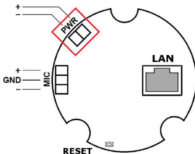
Připojení napájení
